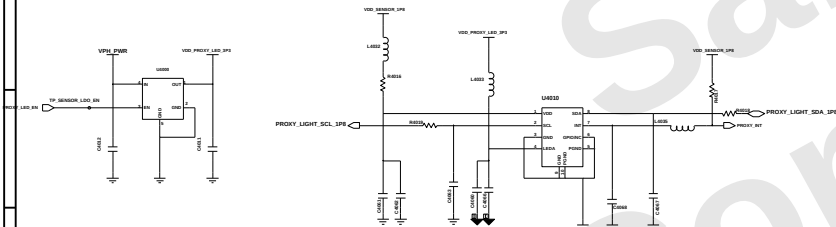
PROXY AMBIENT
