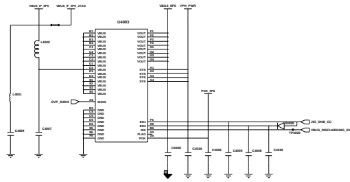
OVP LS
