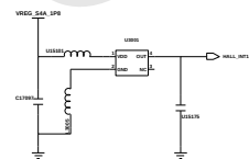
HALL_IC
